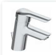
HANSAVANTIS* Waschtisch-Einhand-Einlochbatterie, DN 15 5240 2273 verchromt Ablaufgarnitur (Metall), Anschluss über flexible Druckschläuche G 3/8 Ausladung: 102 mm HANSAVANTIS STYLE 5240 2277 verchromt
